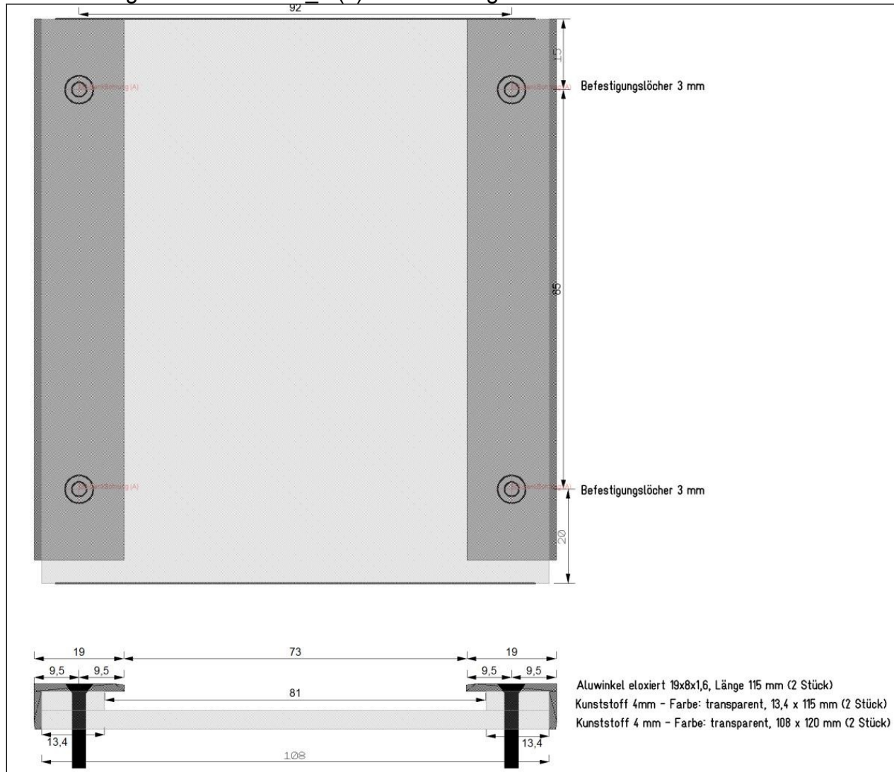
Zeichnung Fassungsboxhalter
