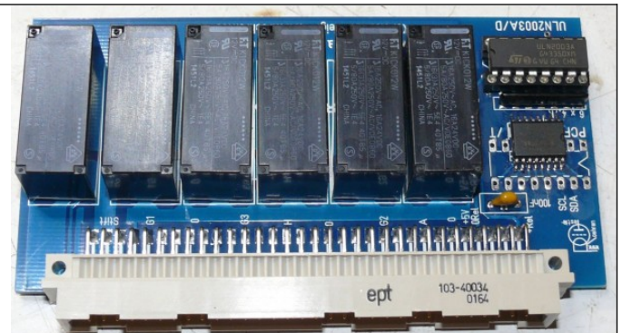
SMD-Version (Bild älterer Leiterplatte)
