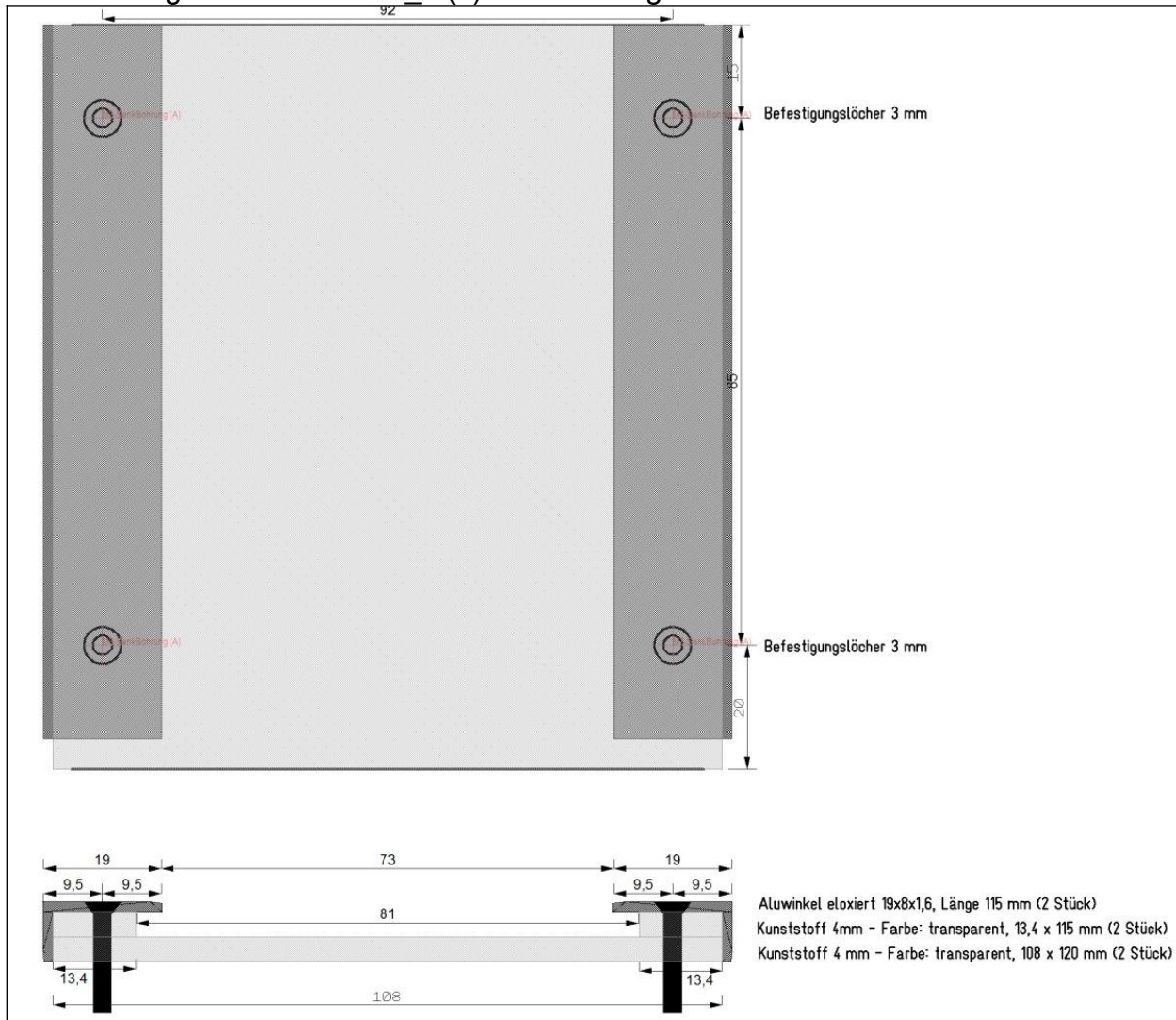
Zeichnung Fassungsboxhalter
